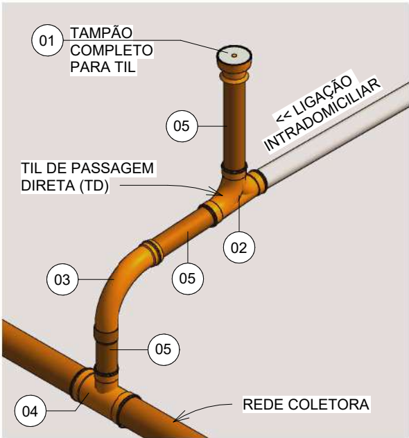
VISTA DA MONTAGEM ESC.:1:25
