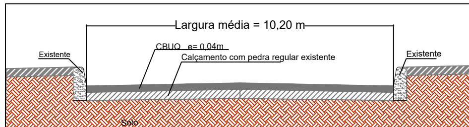
Seção Tipo - Rua Cel. Selbach
