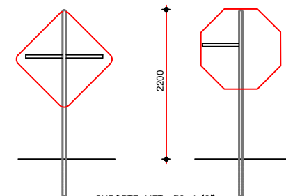
SUPORTE MET. Ø2 1/2" TRAVESSA 1000 x 50 OBSERVAÇÃO : DIMENSÕES EM MILÍMETROS
