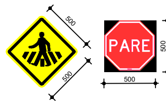
L= 500 P/ VELOCIDADES INFERIORES A 80 km/h OBSERVAÇÃO : DIMENSÕES EM MILÍMETROS
