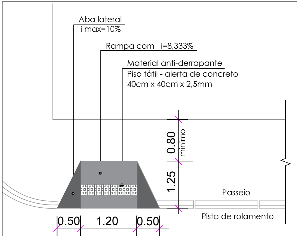
DETALHE : RAMPA DE ACESSO A CADEIRANTES SEM ESCALA
